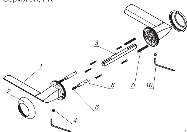
Разнесённый вид дверной ручки
