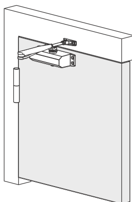
Стандартная установка на полотно для левой двери
