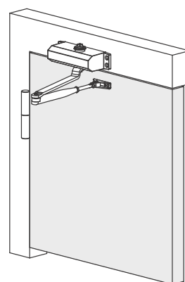
Верхняя установка на короб для левой двери
