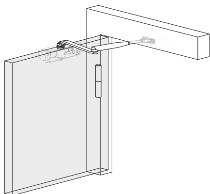
Параллельная установка для левой двери
