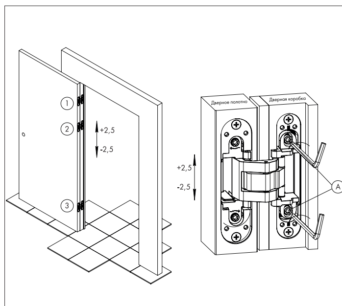
Рисунок 3 — Вертикальная регулировка.
