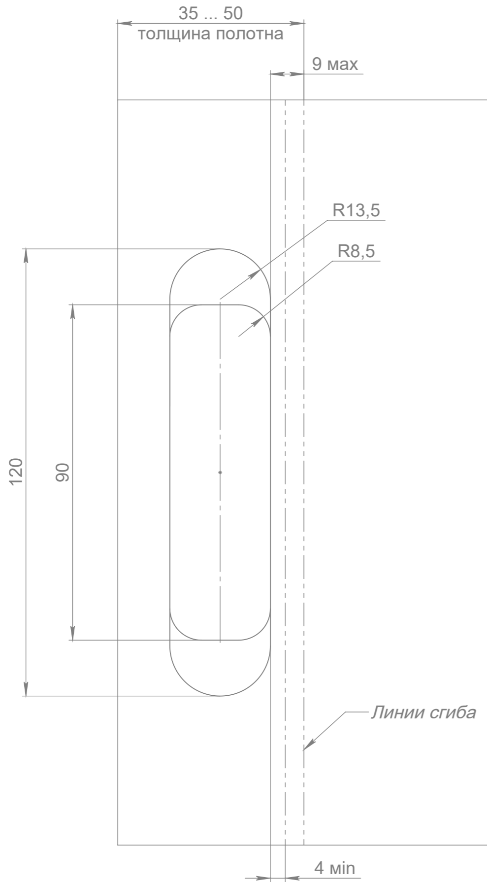
Дверное полотно
